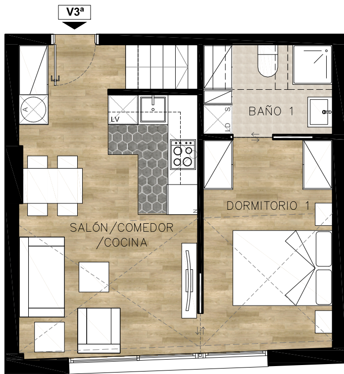
NIVEL 6 PLANTA ACCESO
