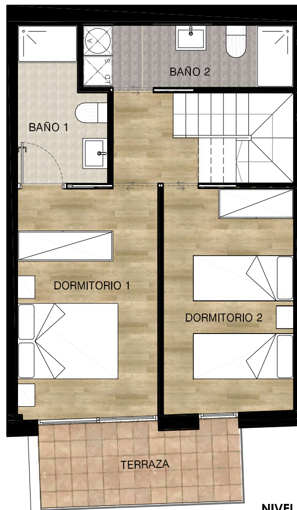
NIVEL 7 PLANTA DUPLEX
